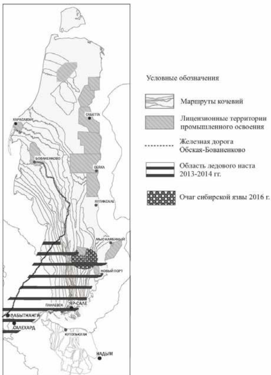
Рис. Полуостров Ямал: масштабы промышленного развития региона на фоне традиционных кочевых маршрутов оленей, а также климатических и эпидемиологических бедствий в 2016 г. 36
